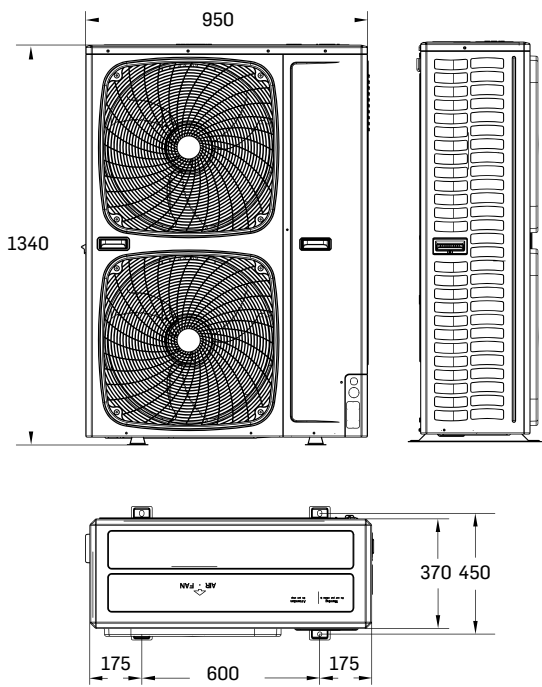
4/5/6 HP Dual Fan Side Discharge
